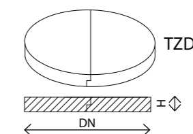
PŁYTA POKRYWOWA DZIELONA
