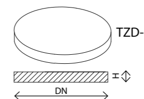
PŁYTA POKRYWOWA PEŁNA
