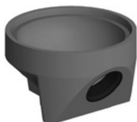
Jest to dno z odpływem/wylotem, służące do odprowadzania wody deszczowej z odpływu. Połączenia rurowe dostępne są dla DN150 i DN200.
